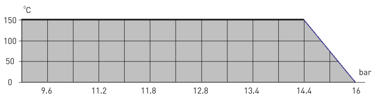
Opseg upotrebljivosti armature PN16
