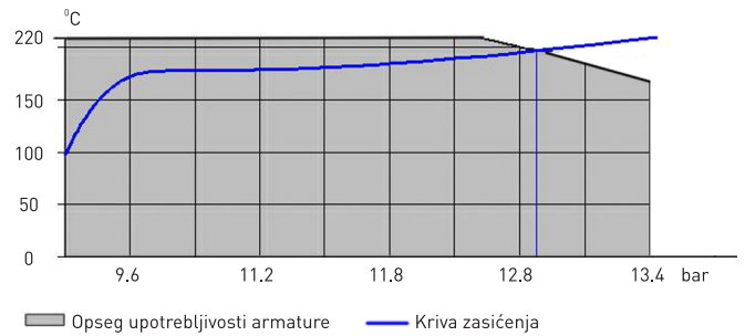
Opseg primene VST ventila sigurnosti, PN16 za prirubničke veze prema EN 1092-2
