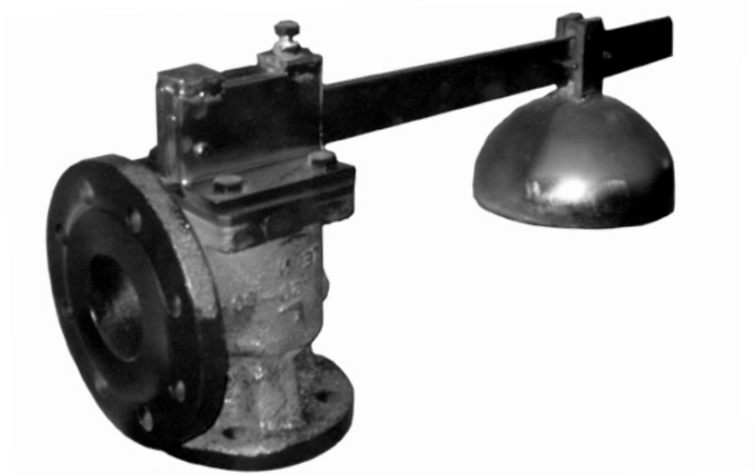
Opseg primene VST ventila sigurnosti, PN16 za prirubničke veze prema EN 1092-2
